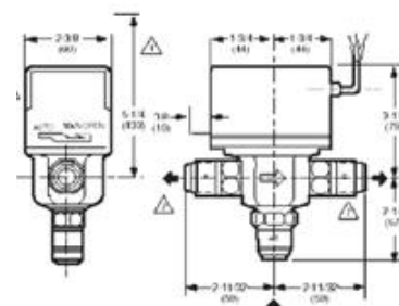
V4044扩口
