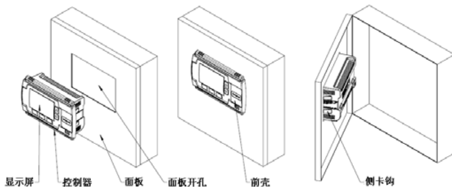
图2 面板安装
