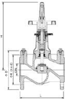
图1 Kombi-SV DN65-DN80
