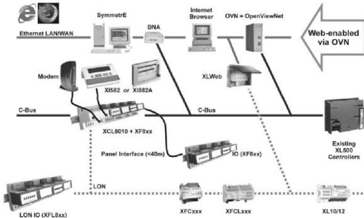
图1.系统结构图
