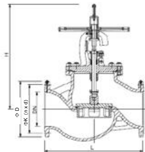
图3 Kombi-SV DN250-DN350
