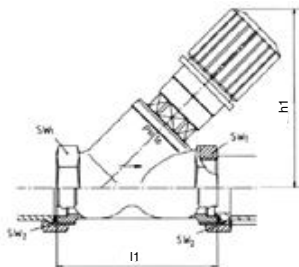
红阀 (V5000)
