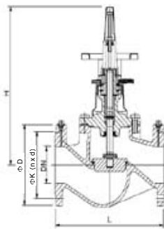
图2 Kombi-SV DN100-DN200
