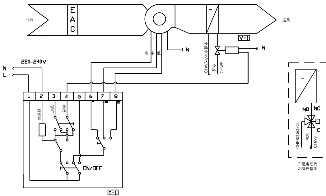
风机盘管控制三 (二管制，单冷/单热水盘管)
