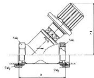
蓝阀 (V5010)
