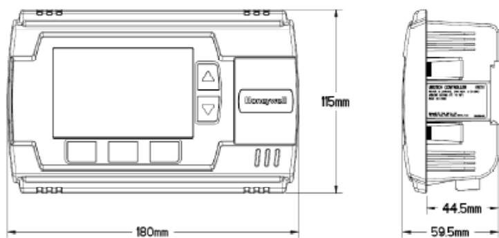
图1 产品尺寸
